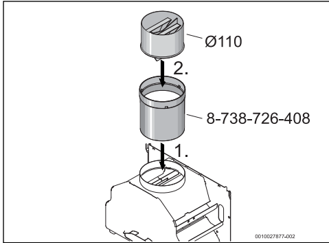
Bild 10 Ø 110 mm montieren
