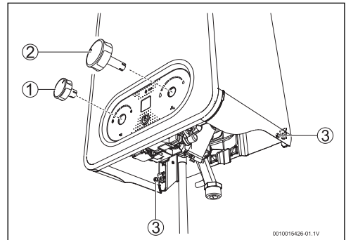
Bild 15 Verkleidung entfernen.
