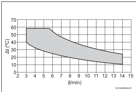
Bild 26 14-Liter-Modell
