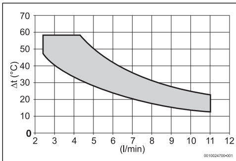
Bild 25 10-Liter-Modell
