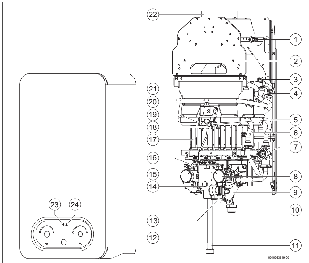
Bild 2 Geräteübersicht
