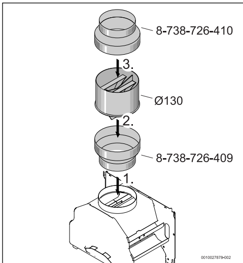
Bild 11 Ø 130 mm montieren
