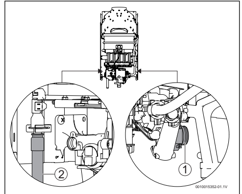
Bild 12 Wasseranschluss
