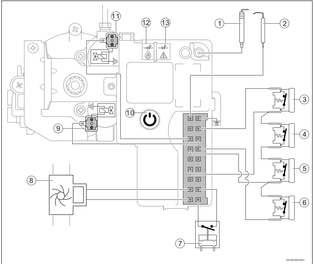
Bild 24 Schaltplan
