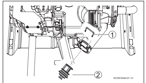
Bild 8 Entleeren
