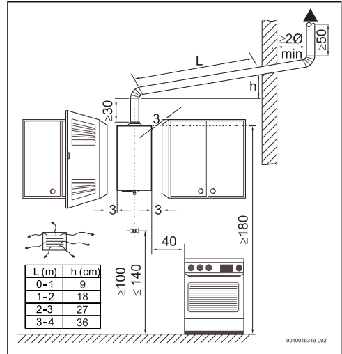
Bild 9 Mindestabstände (cm)
