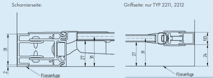
Einbausituation Bodenmontage: (Sondermaß, wenn außerhalb des Produktmaßes) TYP 2211, 2212, 2213, 2214, 2217, 2218
