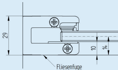
Einbausituation Bodenmontage: (Sondermaß, wenn außerhalb des Produktmaßes) TYP 2215
