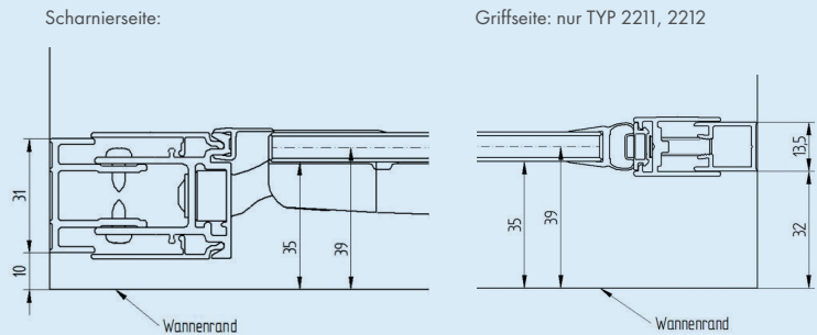
Einbausituation Bodenmontage: (Sondermaß, wenn außerhalb des Produktmaßes) TYP 2211, 2212, 2213, 2214, 2217, 2218
