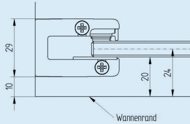
Einbausituation Wannenmontage: TYP 2215
