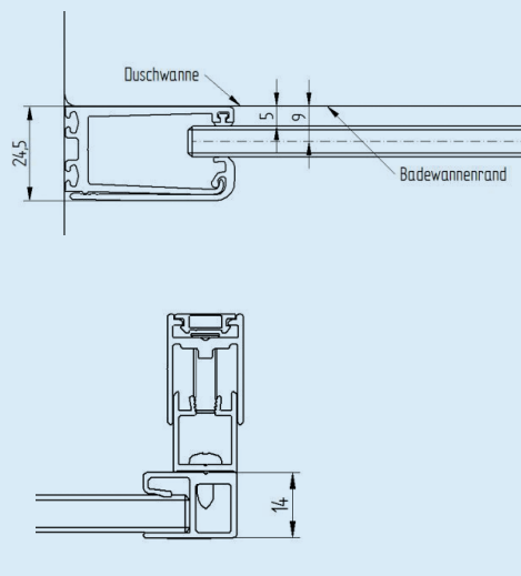
Montage auf Badewanne: TYP 2216
